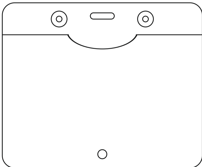
Modell 302 Yttermått ca 110 x 91 mm Innermått ca 108 x 70 mm
