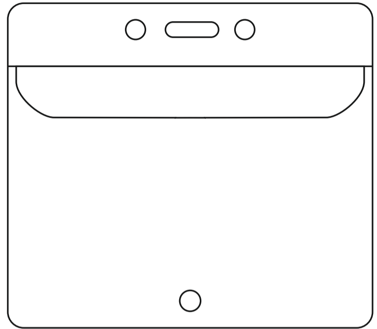
Modell 110 Yttermått ca 98 x 87 mm Innermått ca 95 x 65 mm
